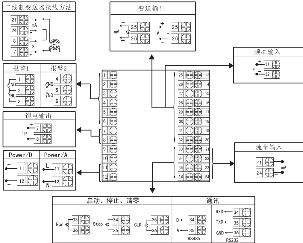
OHR-F661接线图
