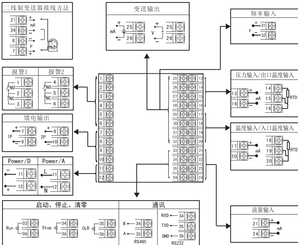
OHR-F662/F663接线图
